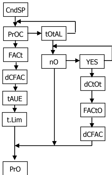
Diagramme de programmation de L’AFFICHAGE en mode: FRÉQUENCEMÈTRE/ TACHYMÈTRE
